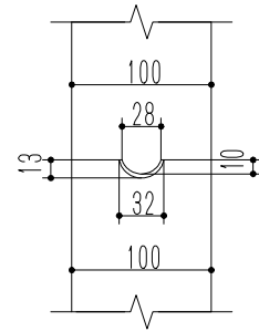
a部詳細
